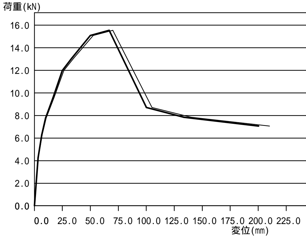
2 階 Y 方向 X10' 9.100m 荷重-変形関係曲線(ねじれ補正後 補正值= 1.0484)
