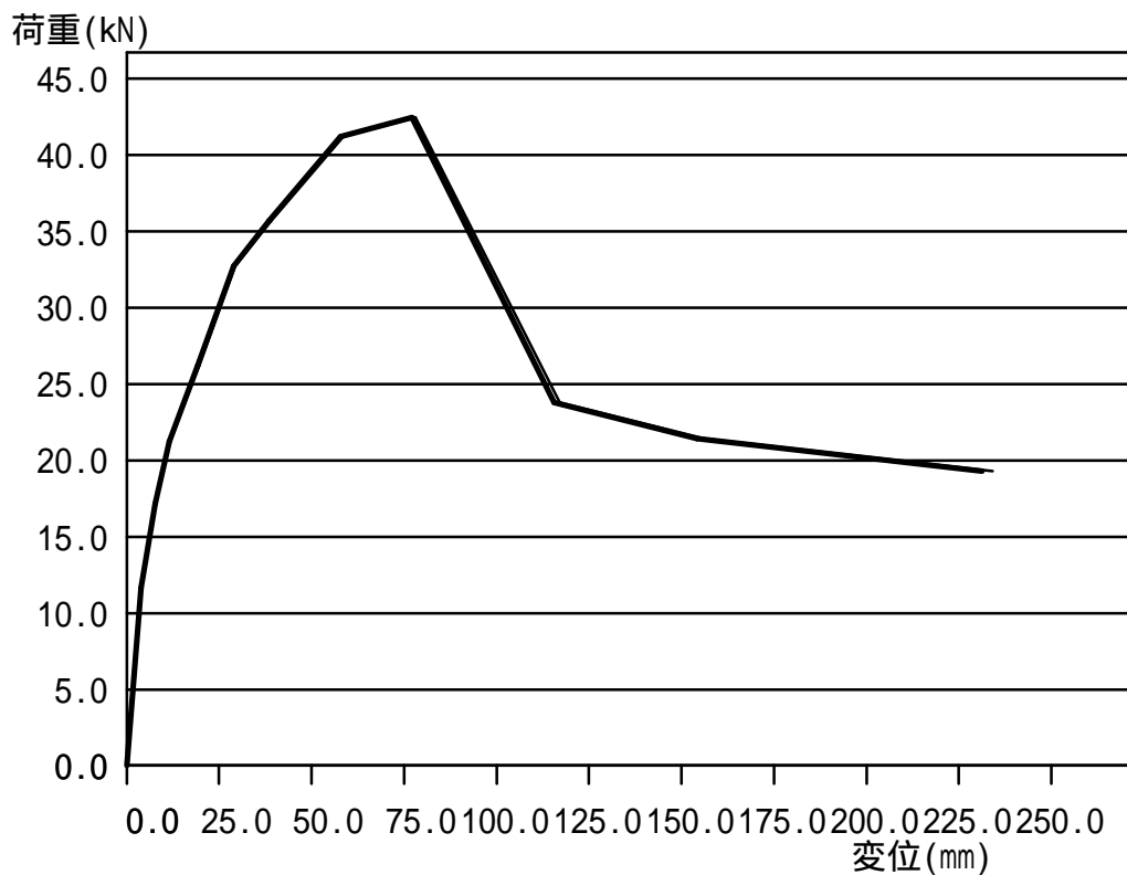
1 階 Y 方向 X11 9.470m 荷重-変形関係曲線(ねじれ補正後 補正值= 1.0116)
