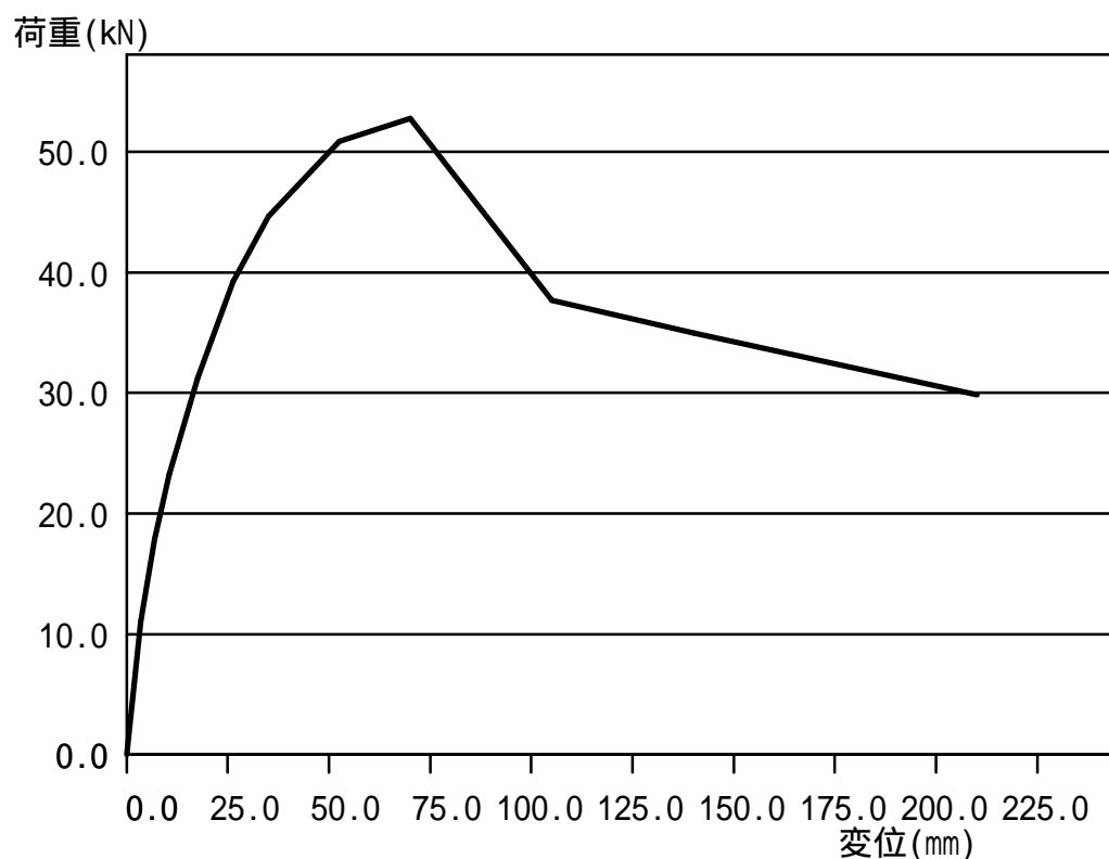
2階 方向 Y1 0.000m 荷重-変形関係曲線
