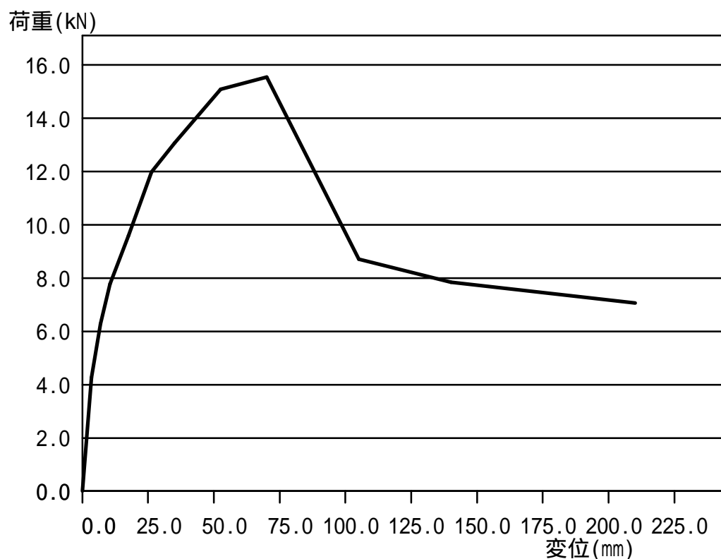
2階 Y方向 X10' 9.100m 荷重-変形関係曲線
