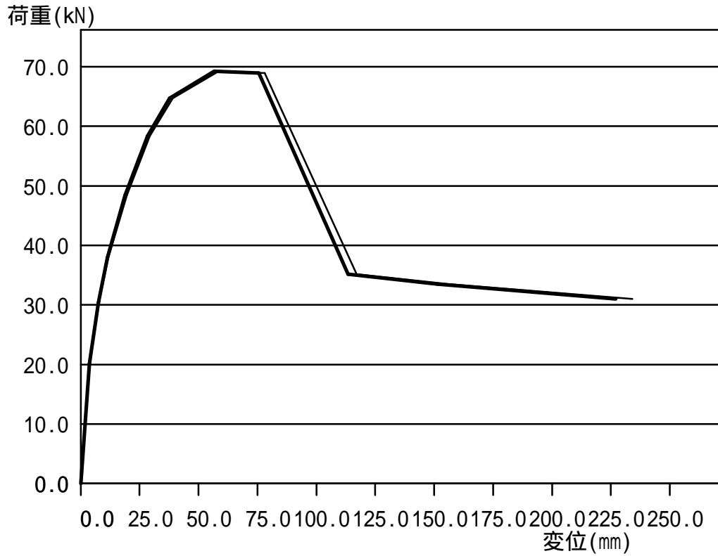
1 階 Y 方向 X1 0.000m 荷重-変形関係曲線(ねじれ補正後 補正值= 1.0306)
