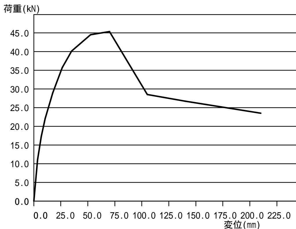
2階 方向 Y11 9.555m 荷重-変形関係曲線
