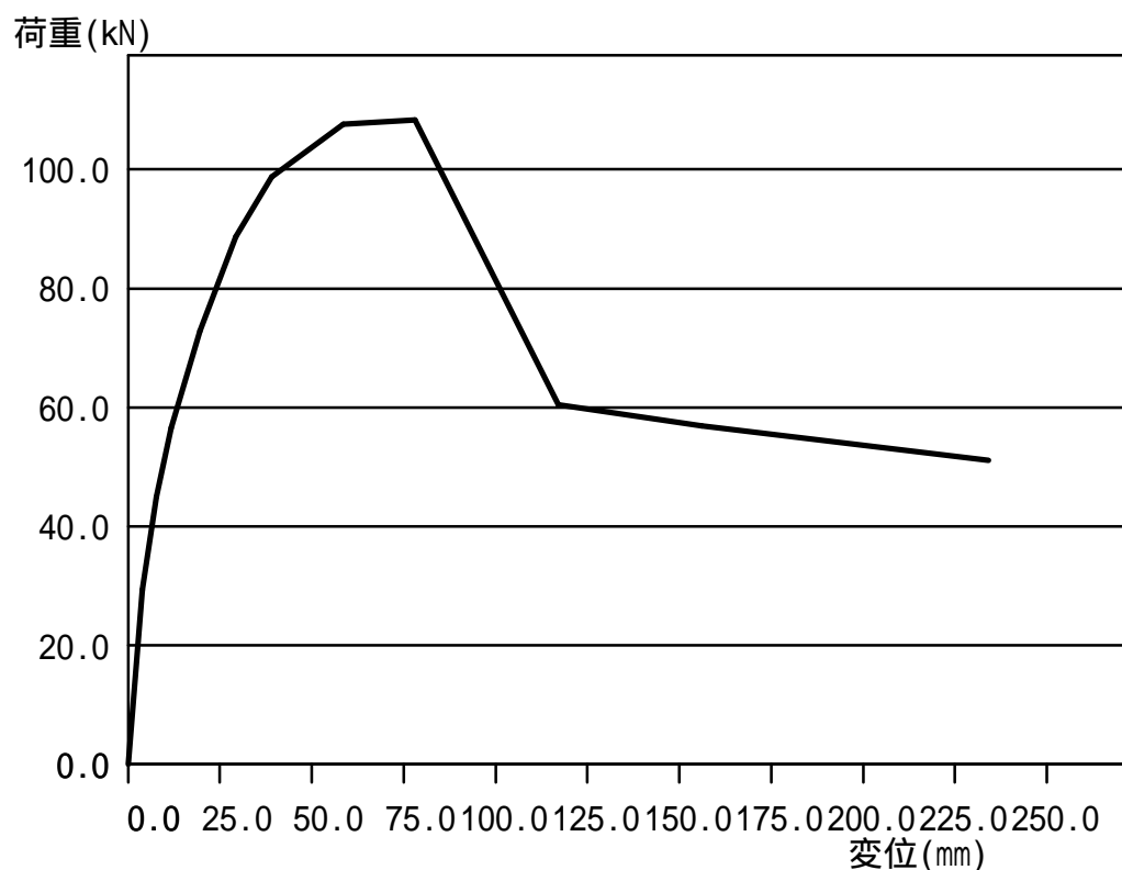
1階 方向 Y11 9.555m 荷重-変形関係曲線
