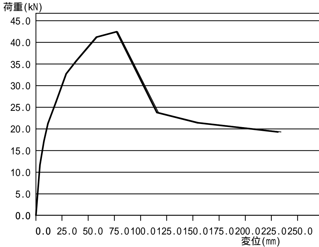
1 階 Y 方向 X10' 9.100m 荷重-変形関係曲線(ねじれ補正後 補正值= 1.0123)
